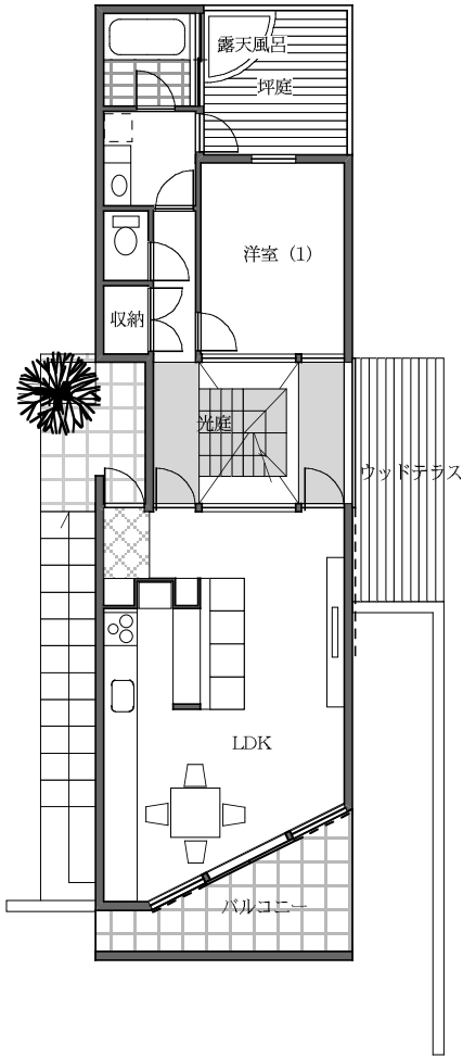
1階平面図
