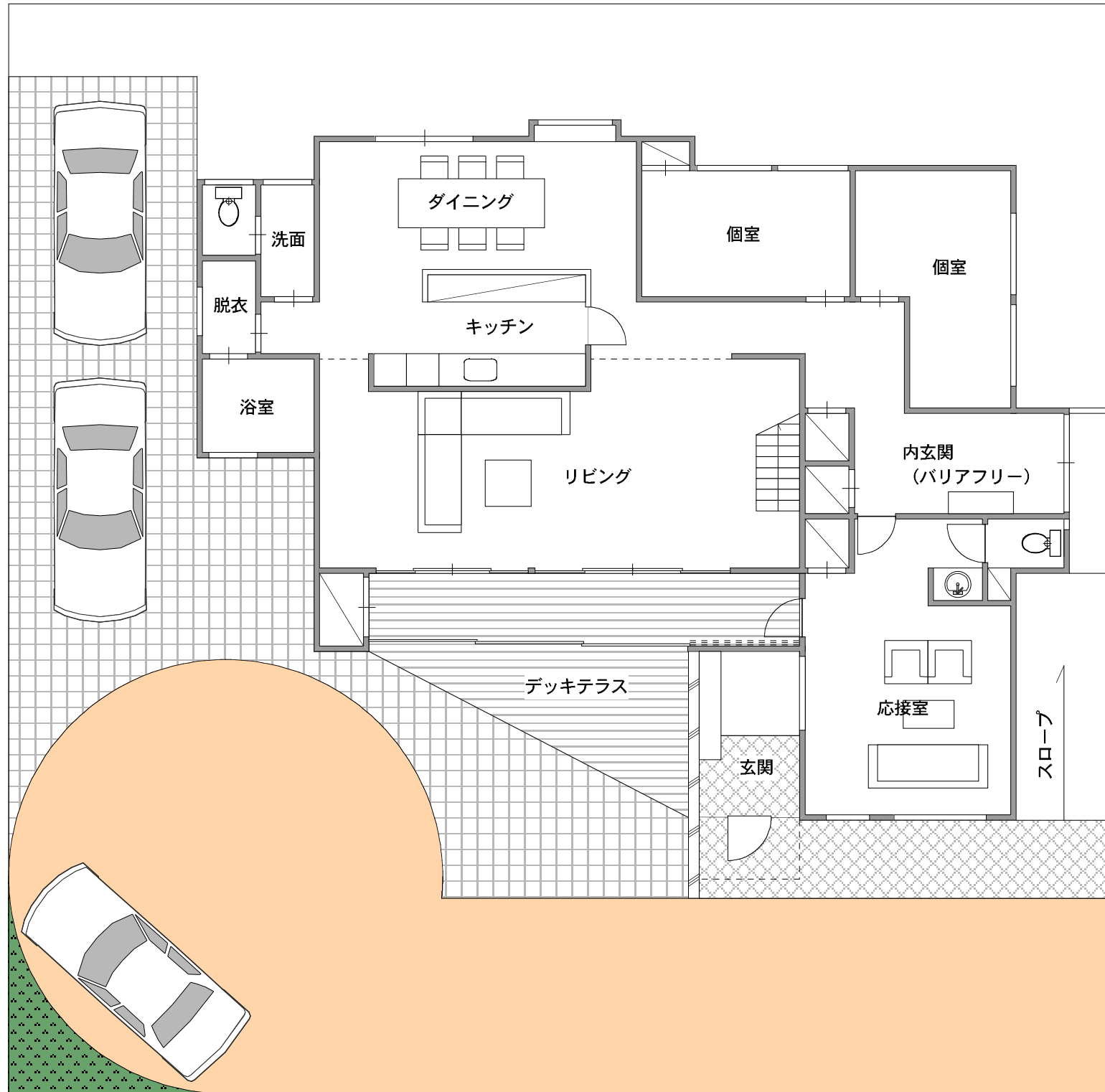
配置図兼1階平面図
